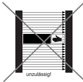
Bild 25.2 Ortsfeste oder -variable Ausblendung mit teilweiser Abdeckung des ausgeblendeten Teils des Lichtvorhanges. Zusätzliche Abdeckung erforderlich!
