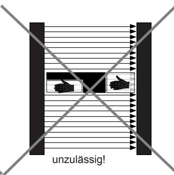
Bild 25.3 Ortsfeste oder -variable Ausblendung mit teilweiser Abdeckung des ausgeblendeten Teils des Lichtvorhanges. Zusätzliche Abdeckungen erforderlich!
