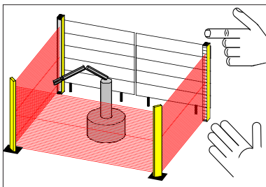
Bild 4/4 Absicherung von Zugangsbereichen über Umlenkspiegel
