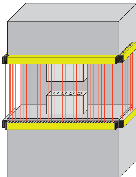
Absicherung einer C-Press auf 3 Seiten ohne Behinderung durch senkrechte Umlenksiegel.
