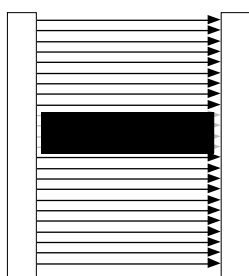
Bild 25.1 Ortsfeste oder -variable Ausblendung mit kompletter Abdeckung des ausgeblendeten Teils des Lichtvorhangs.
