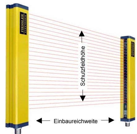
Bild 35/1 Einbaureichweite , Hindernisgroe, Schutzfeldhoe
