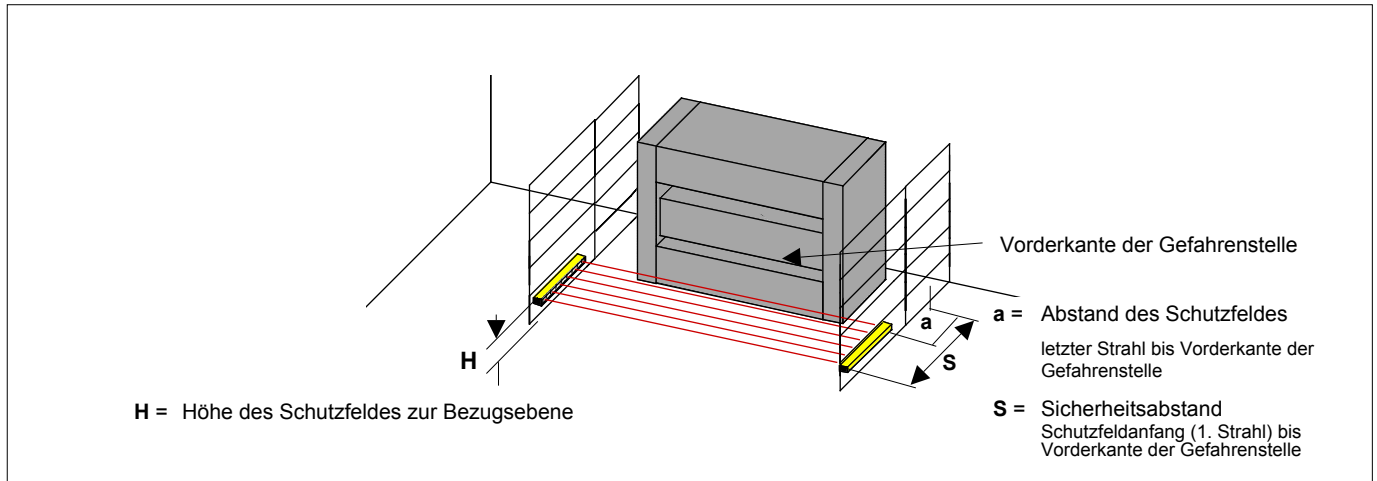
Bild 13/1 Horizontale Absicherung
