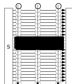
Bild 25.4 Durchfahren des Schutzfeldes mit entsprechendem Prüfstab
