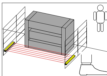
Bild 4/2 Bereichsabsicherung
