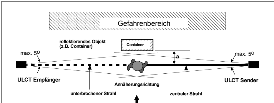
Bild 14/1 Abstand zu spiegelnden Flächen
