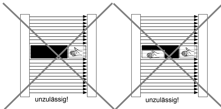
Bild 25.2 Ortsfeste oder -variable Ausblendung mit teilweiser Abdeckung des ausgeblendeten Teils des Lichtvorhangs. Zusätzliche Abdeckung erforderlich!
