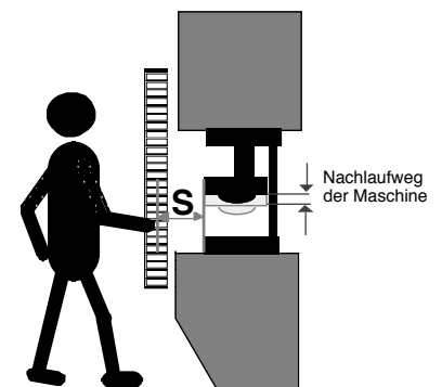
Bild 35/2 Sicherheitsabstand u. Nachlaufweg
