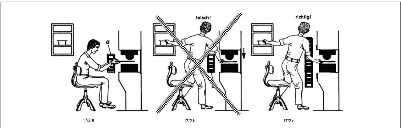
Bild 17/2a,b,c Schutz gegen Untergreifen und Übergreifen
