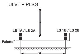
Für ein einwandfreies Funktionieren der Überbrückung muss S kleiner oder gleich sein, wie die Länge der Palette.
