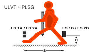
Gegebenenfalls muss der Abstand H zur begehbaren Fläche oder der Abstand S vergrößert werden.
