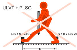
Der Abstand S muss so groß sein, dass ein gleichzeitiges Unterbrechen der Mutingsensoren LS 1A/LS 2A und LS 1B/LS 2B durch einen Menschen nicht möglich ist.
