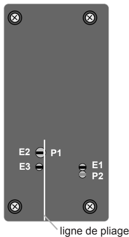
Vue des fenêtres des récepteurs
