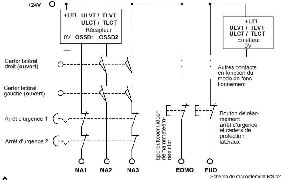
Schéma de raccordement 6/S.42
