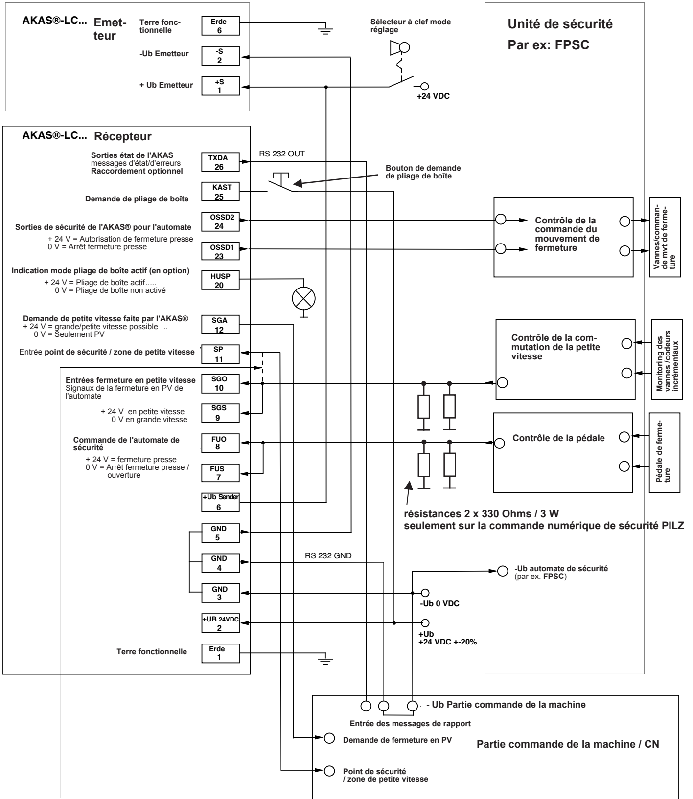
Schéma de raccordement 0/S.35
