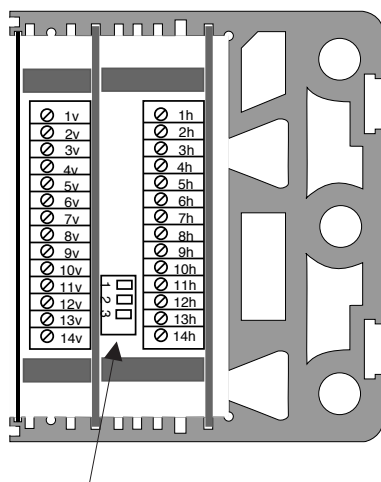
Borniers de raccordement AKAS®-3F / -IIF Récepteur
