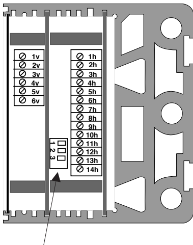
Borniers de raccordement Récepteur
