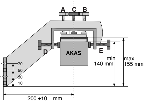
Dessin, vue de dessus Fig. 18/3
