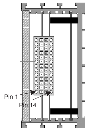
Vue de coté après retrait du capot latéral du boîtier récepteur
