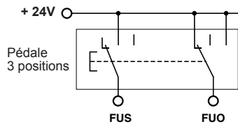
Schéma de raccordement 4a/S.40
