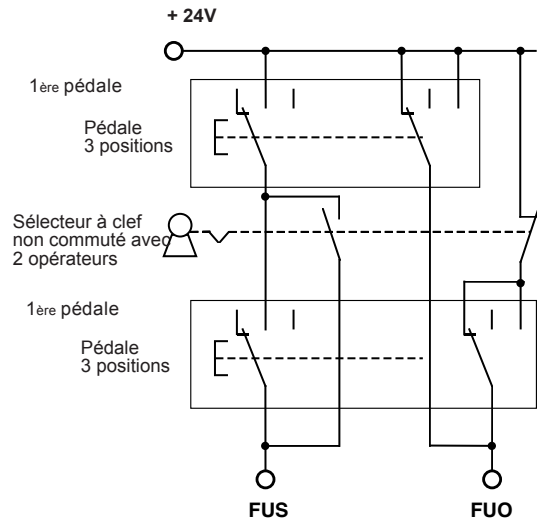
Schéma de raccordement 4b/S.40
