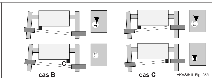
Ajustement non correct de l'émetteur
