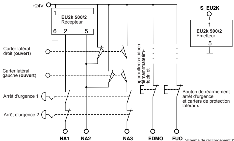
Schéma de raccordement 7/S.42
