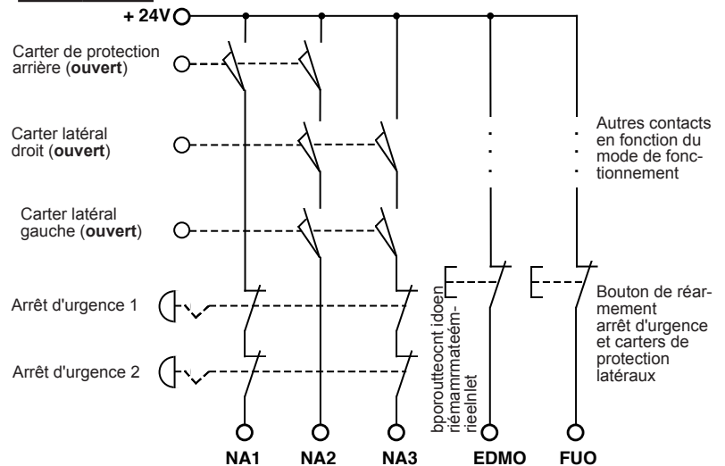
Schéma de raccordement 5b/S.41
