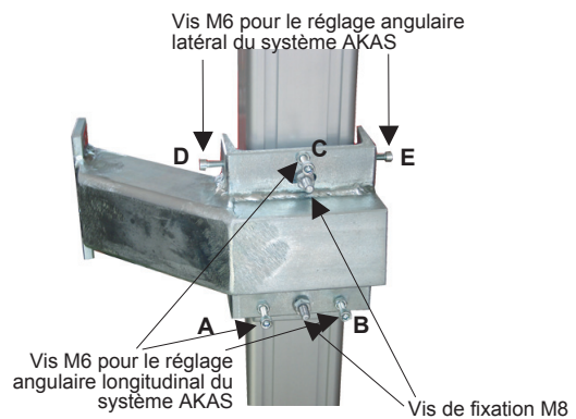
Vue arrière du support Fiesler fig. 21/3
