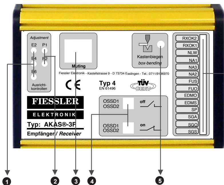
Vue des fenêtres des récepteurs
