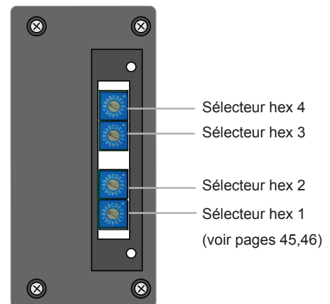
Vue de coté après retrait du capot latéral du boîtier récepteur
