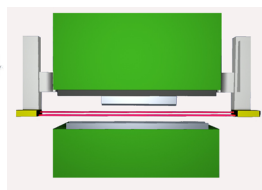
Système de protection AKAS pour presses plieuses
