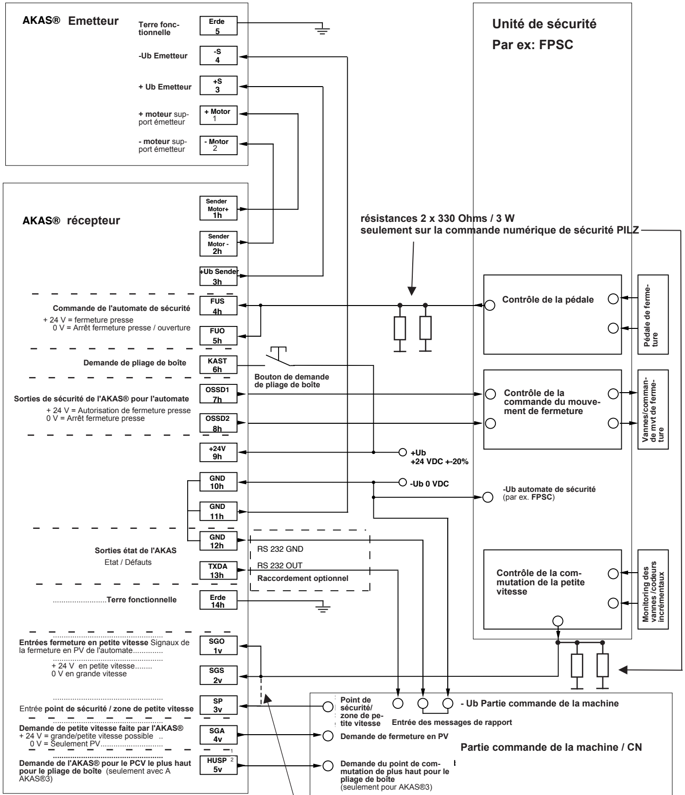
Schéma de raccordement 1/S.33
