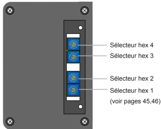
Vue de coté après retrait du capot latéral du boîtier récepteur
