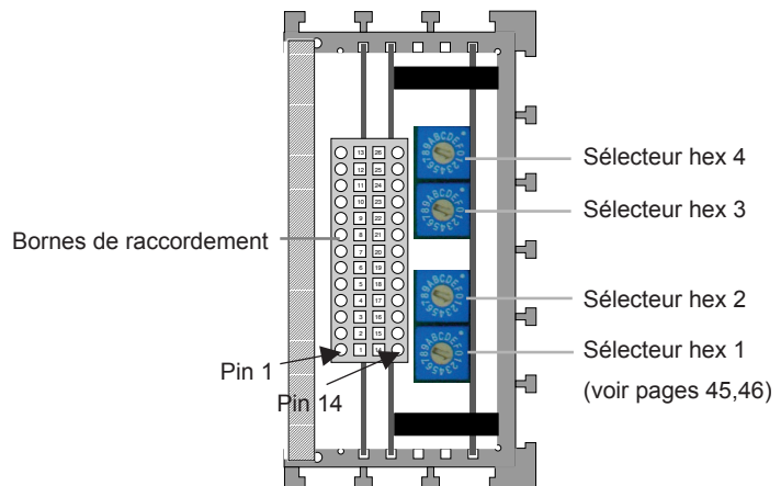
Vue de côté après retrait du capot latéral du boîtier récepteur
