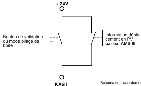
Schéma de raccordement 10/S.44
