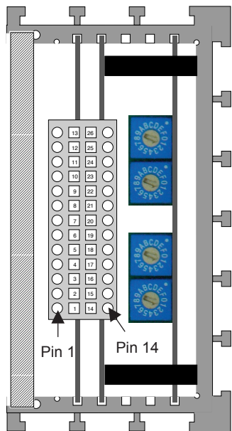
Bornes de raccordement AKAS®-LCF Récepteur
