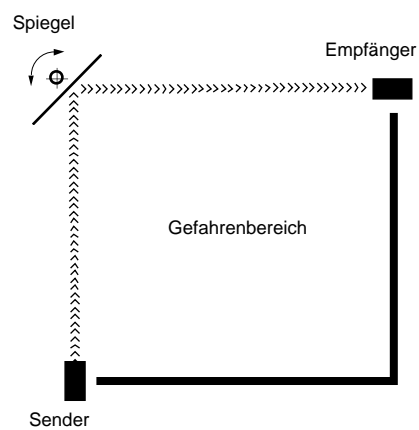
Bild 21/3 Anordnung über 1 Umlenkspiegel
