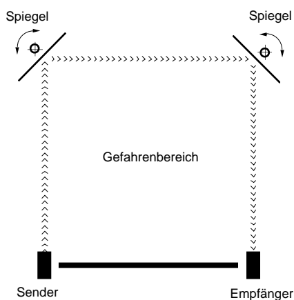
Bild 21/2 Anordnung über 2 Umlenkspiegel
