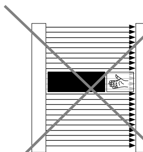
Bild 29.2 Ortsfeste oder -variable Ausblendung mit teilweiser Abdeckung des ausgeblendeten Teils des Lichtvorhanges. Zusätzliche Abdeckung erforderlich!
