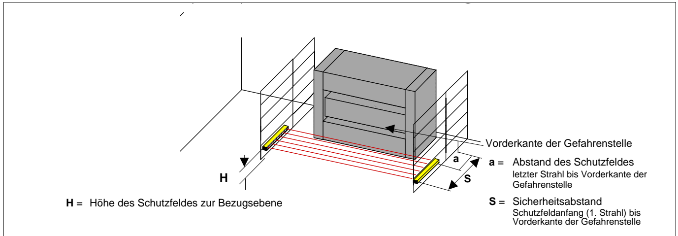
Bild 15/1 Horizontale Absicherung
