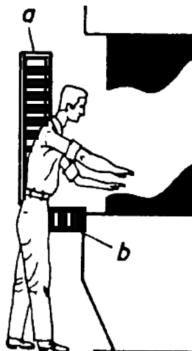
Bild 33/2 Hintertretschutz
