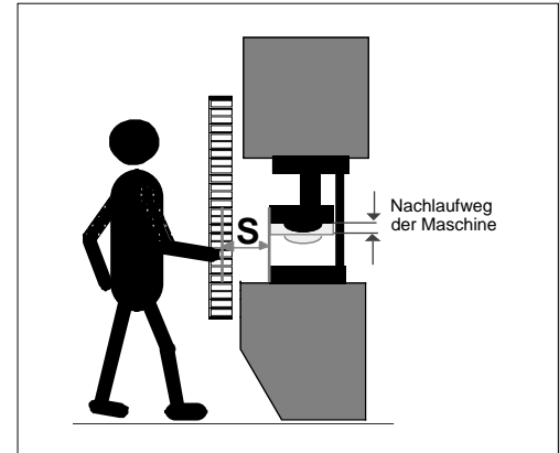
Bild 14/1 Vertikale Gefahrstellenabsicherung
