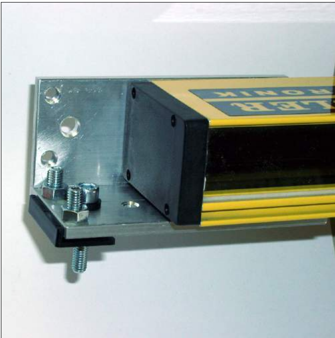
Bild 20/1 montierte Winkellaschen am Lichtvorhang
