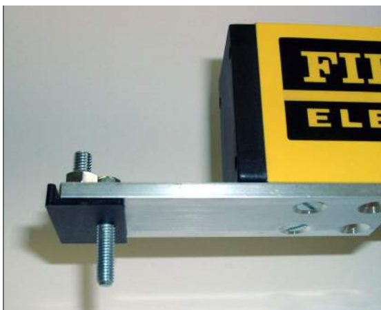
Bild 19/3 montierte Standard-Befestigungslaschen am Lichtvorhang
