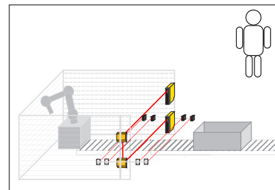
Bild 8/6 Zugangssicherung mit Muting
