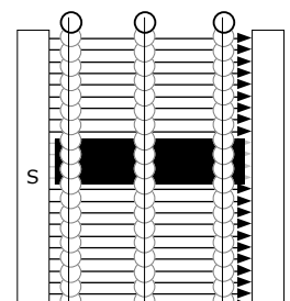
Bild 29.4 Durchfahren des Schutzfeldes mit entsprechendem Prüfstab
