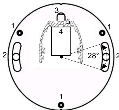
Bild 24/2 Säule mit Lichtvorhang ULVT bzw. BLVT montiert
