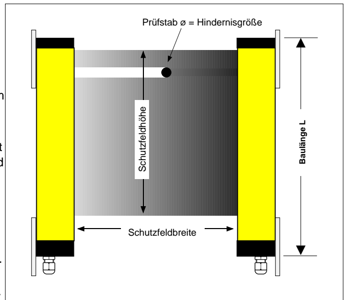
Bild 9/1 Sender und Empfänger bilden das Schutzfeld
