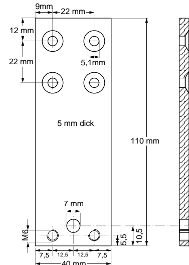
Bild 12/2 Befestigungslaschen
