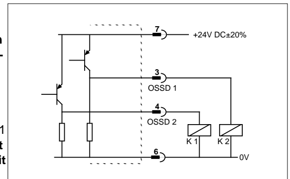
Bild 25/3 Ausgänge 1 und 2
