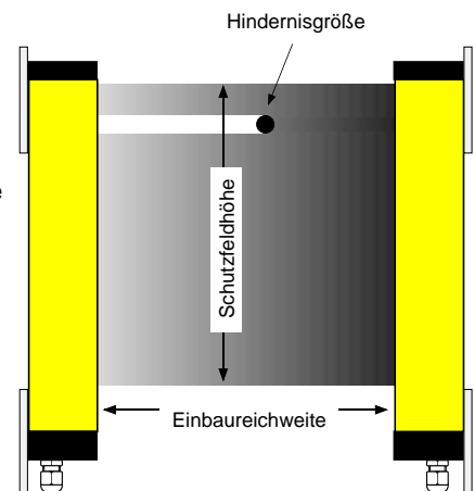
Bild 6/1 Einbaubreite, Hindernisgröße, Schutzfeldhöhe
