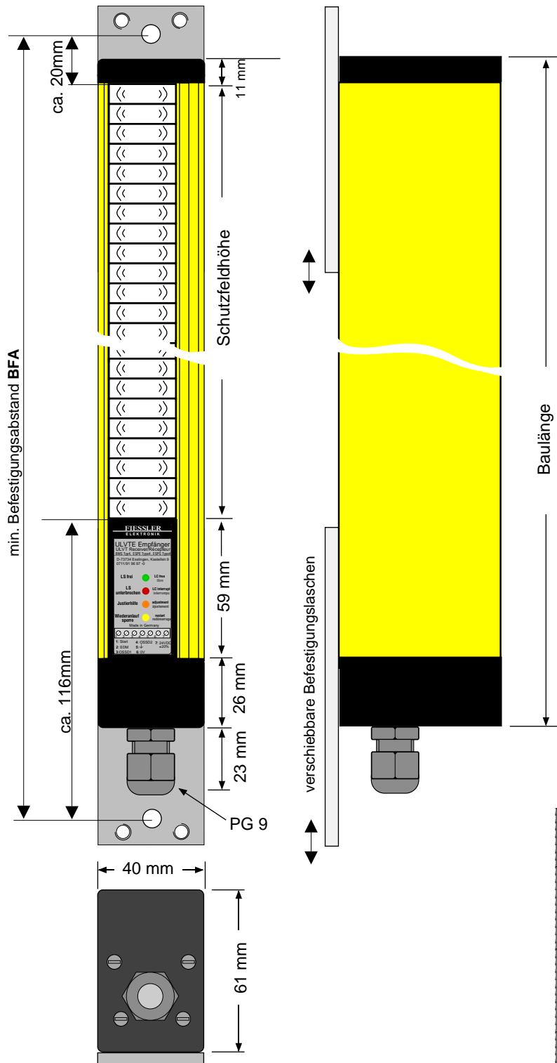
Bild 12/1 Maße Sender / Empfänger
