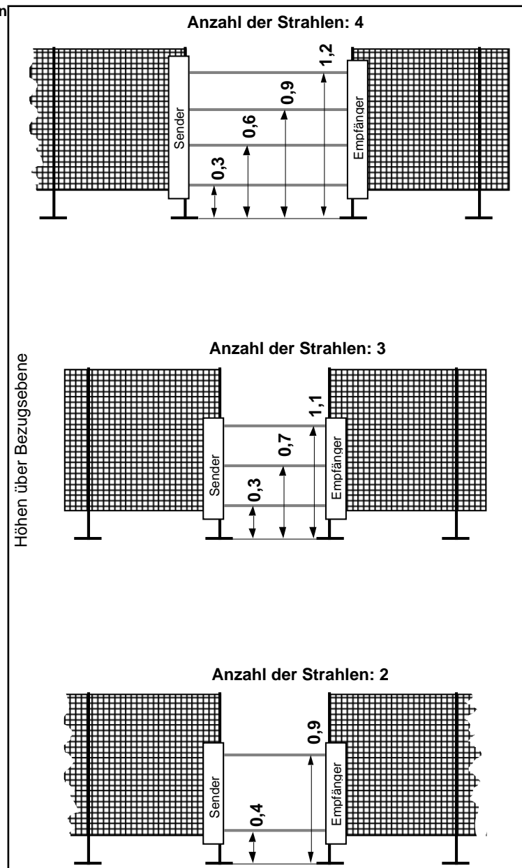
Bild 16/1 Vertikale Absicherung
