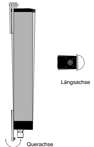
Bild 27/2 Quer-Längsachse
