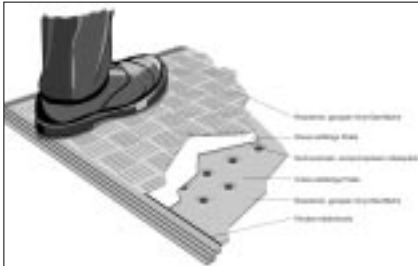
Sicherheits-Schaltmatten
