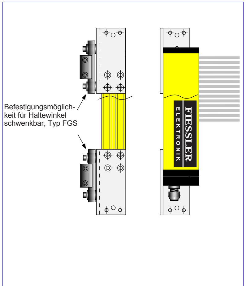
Bild 20/4 Winkellaschen
