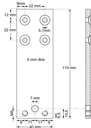
Bild 12/2 Befestigungslaschen
