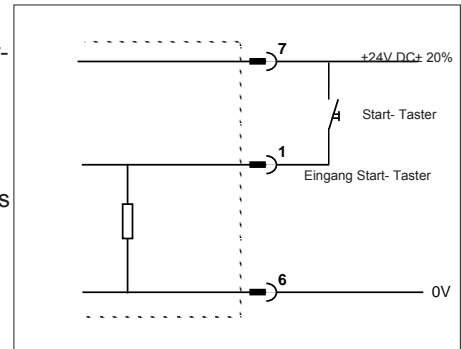
Bild 26/1 Eingang Starttaster
