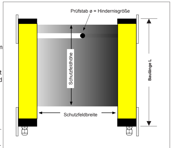
Bild 9/1 Sender und Empfänger bilden das Schutzfeld
