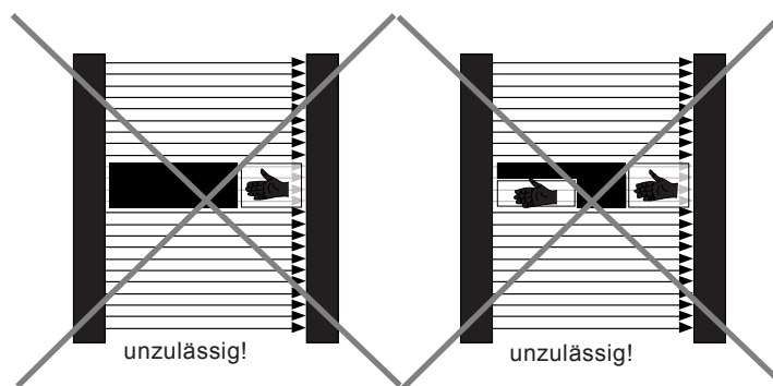
Bild 29.3 Ortsfeste oder -variable Ausblendung mit teilweiser Abdeckung des ausgeblendeten Teils des Lichtvorhanges. Zusätzliche Abdeckungen erforderlich!
