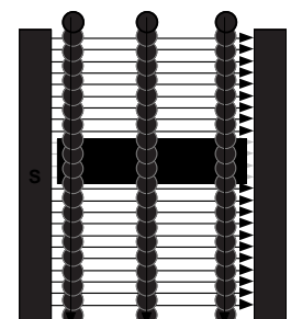
Bild 29.4 Durchfahren des Schutzfeldes mit entsprechendem Prüfstab
