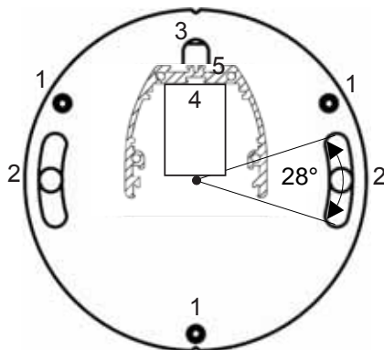
Bild 24/2 Säule mit Lichtvorhang ULVT bzw. BLVT montiert
