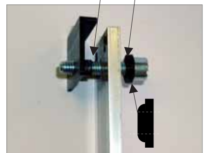
Bild 19/5 Isolierteile montiert
