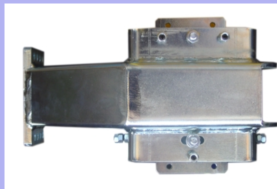
U-Halter mit Justierschrauben
