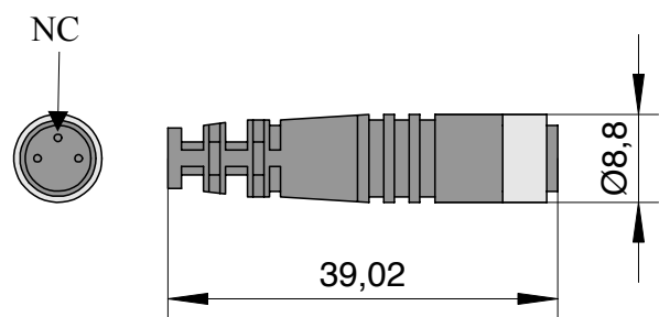
Kupplung M8
