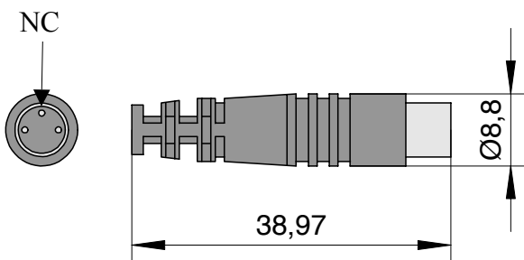
Stecker M8
